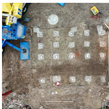
Figuur 26: Sleuf fundering
