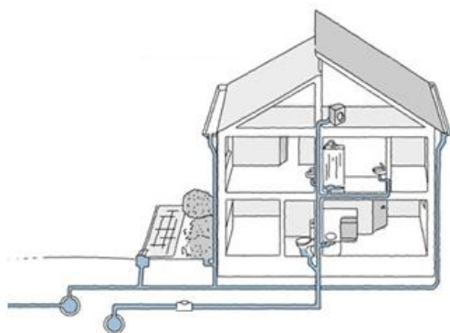
Figuur 27: Gescheiden rioleringsstelsel
