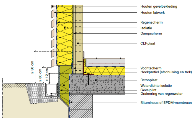
Figuur 28: Drainage
