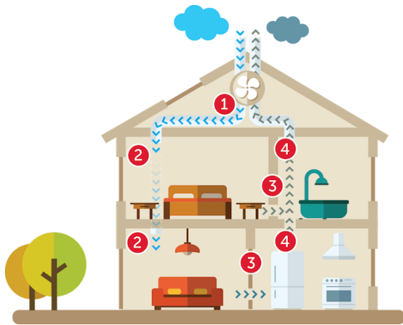
Figuur 21: Ventilatiesysteem D
