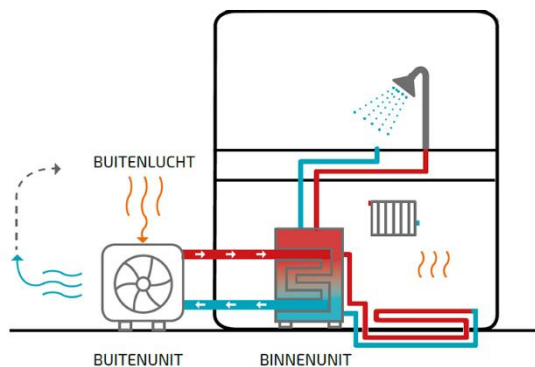
Figuur 18: Lucht/Water Warmtepomp principe
