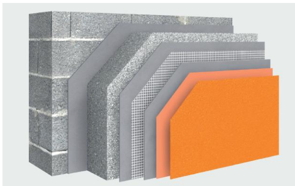
Figuur 8: Crepi + EPS
