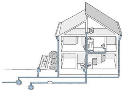
Figuur 28: Gescheiden rioleringsstelsel
