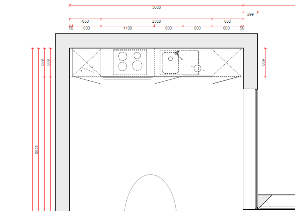
Figuur 18: Grondplan keuken type 1
