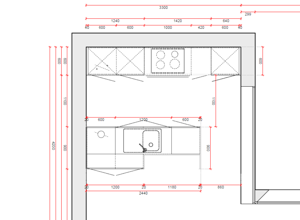
Figuur 20: Grondplan keuken type 2
