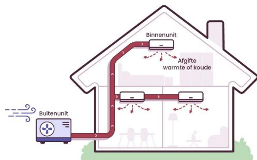
Figuur 24: Lucht/Lucht warmtepomp principe
