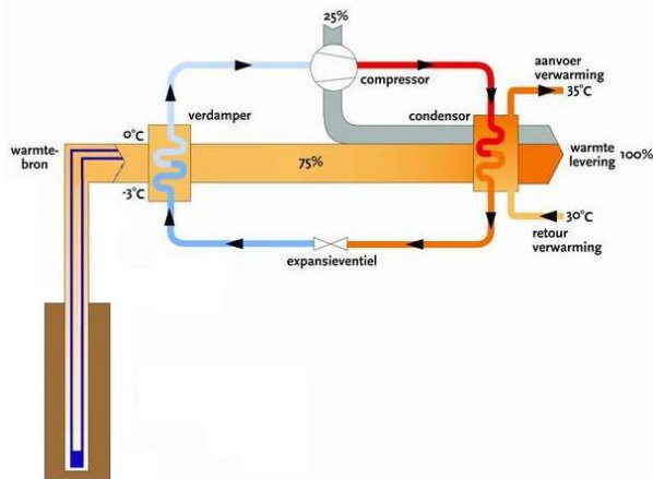
Figuur 26: Geothermische warmtepomp principe
