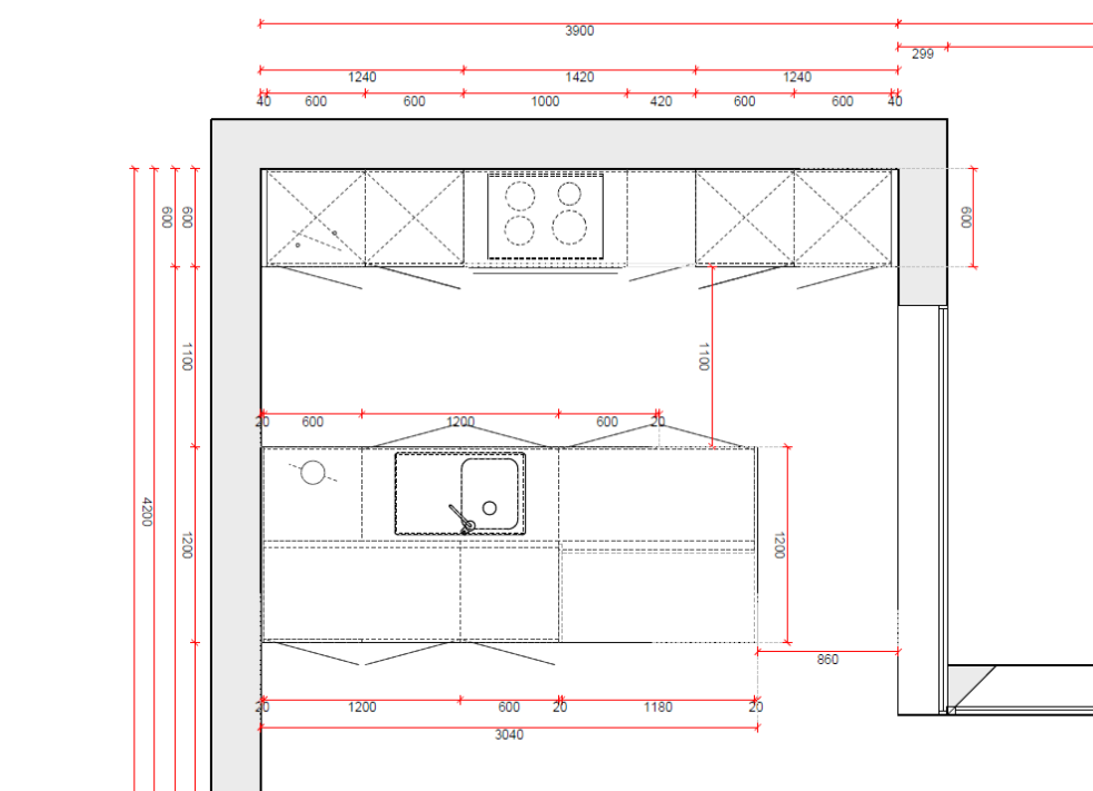
Figuur 22: Grondplan keuken type 3
