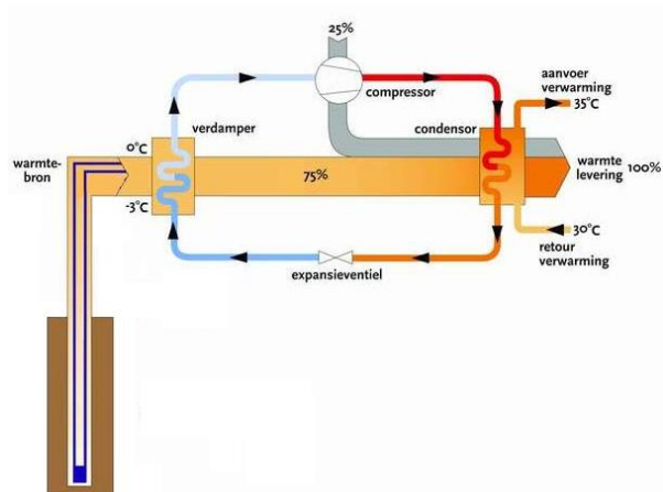
Figuur 27: Geothermische warmtepomp principe
