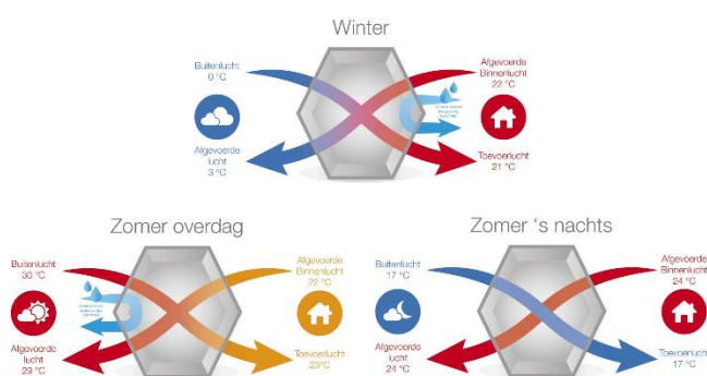
Figuur 29: Regeling enthalpiewisselaar
