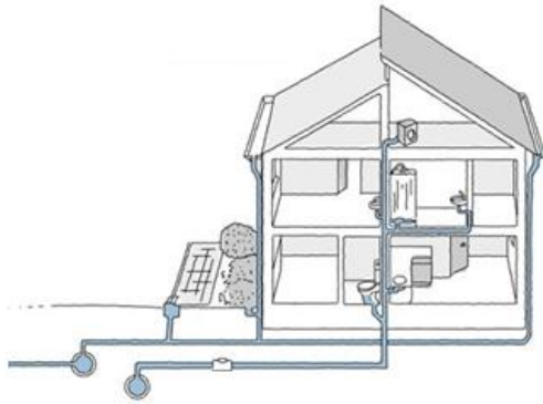
Figuur 38: Gescheiden rioleringsstelsel
