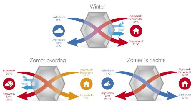
Figuur 32: Regeling enthalpiewisselaar
