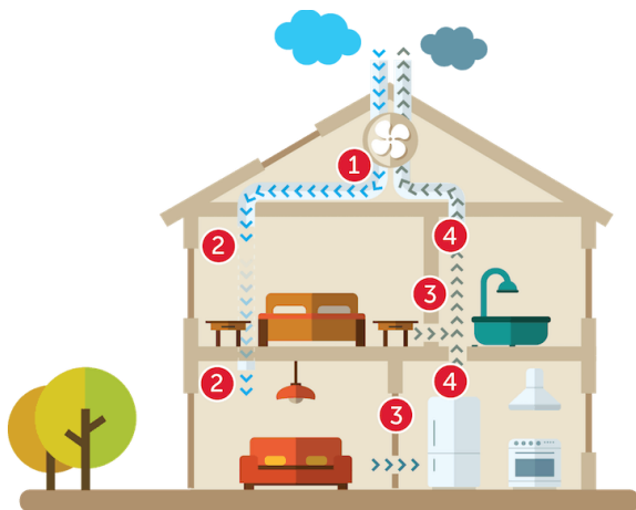
Figuur 31: Ventilatiesysteem D
