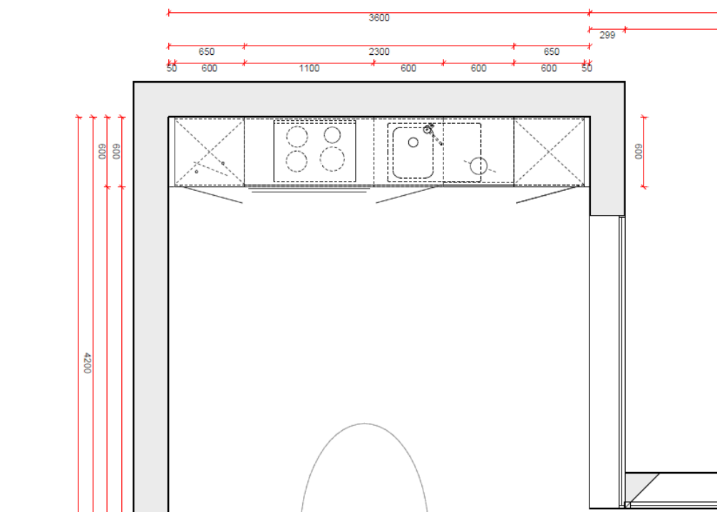
Figuur 21: Grondplan keuken type 1
