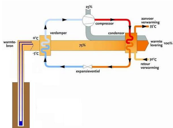
Figuur 30: Geothermische warmtepomp principe
