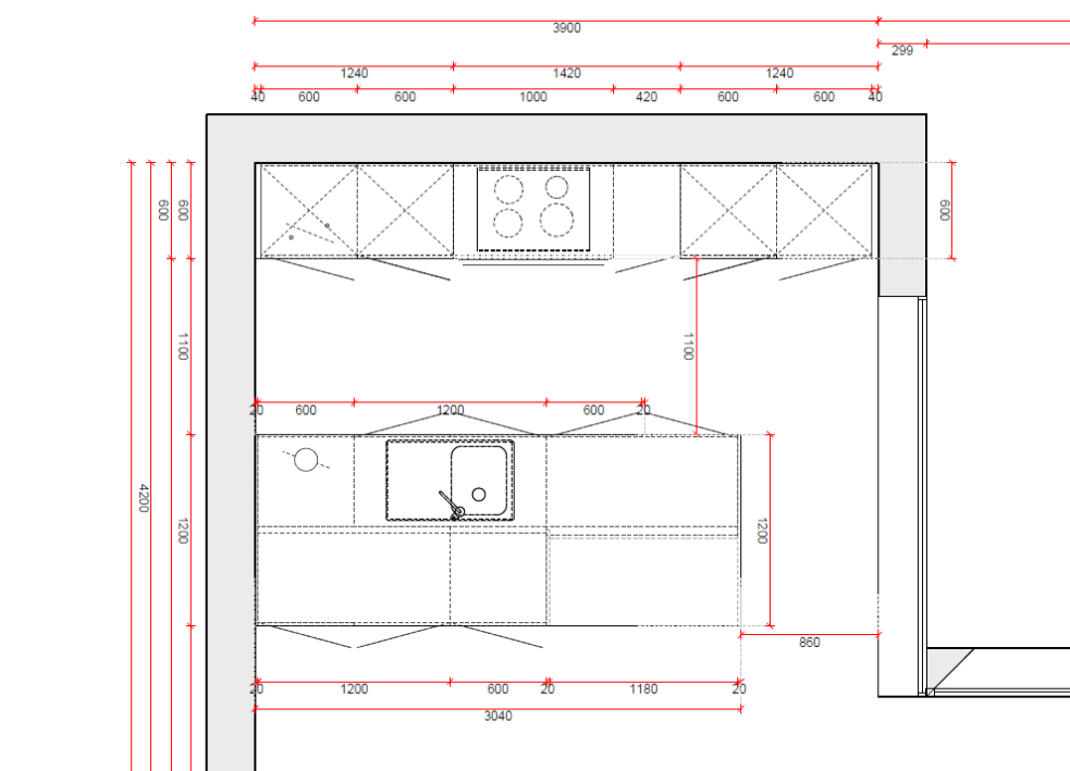
Figuur 25: Grondplan keuken type 3
